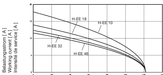
H-EE 10 / 18 / 32 / 46 1,5 mm 2
